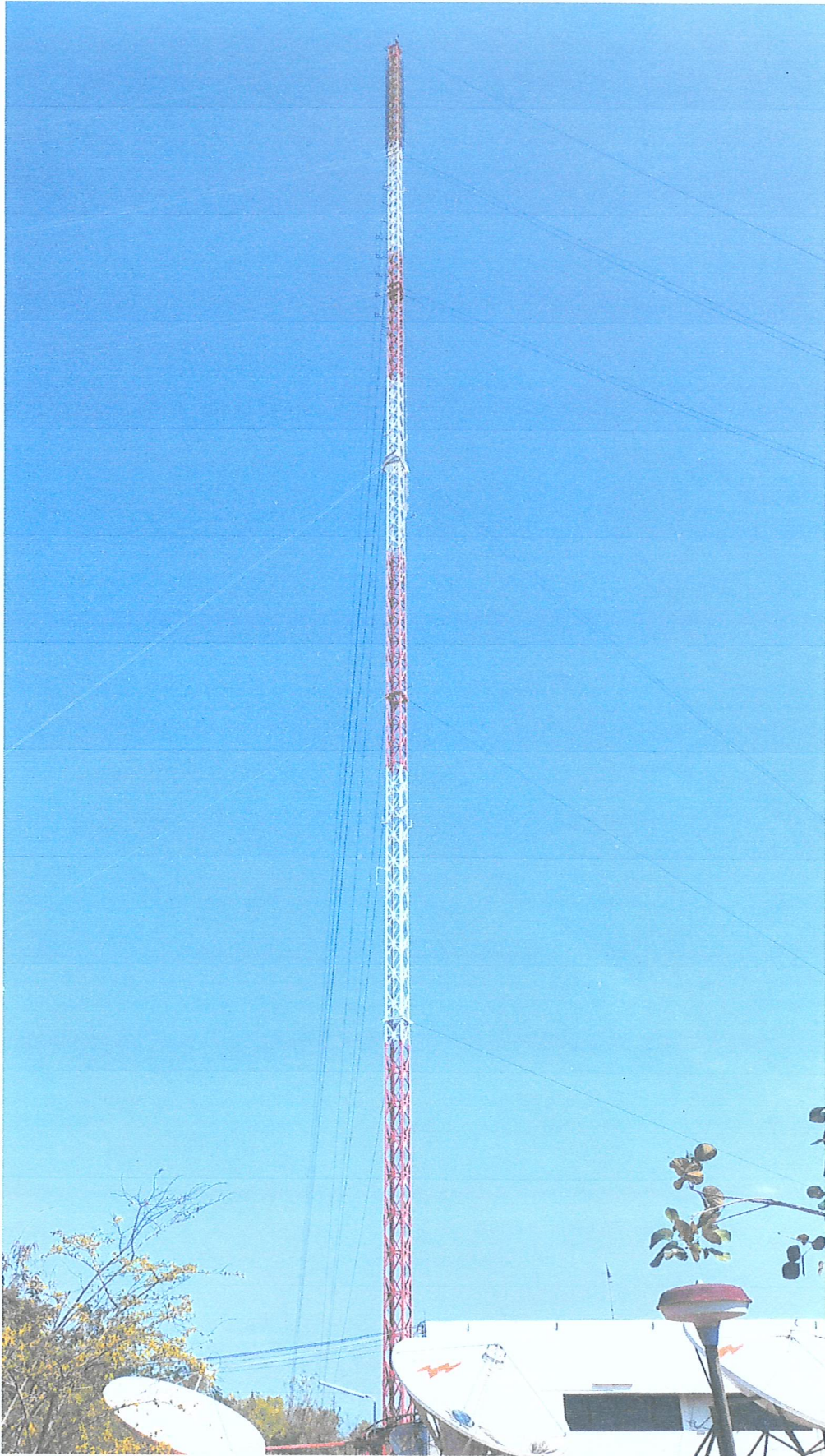
ภาพ : เสาอากาศเครื่องส่งโทรทัศน์ จ.ขอนแก่น ความสูง 150 เมตร
